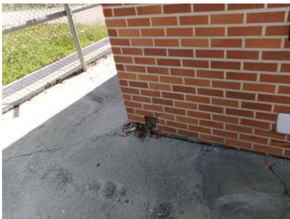
<1~2호지 검수실 외부 조적파손>
