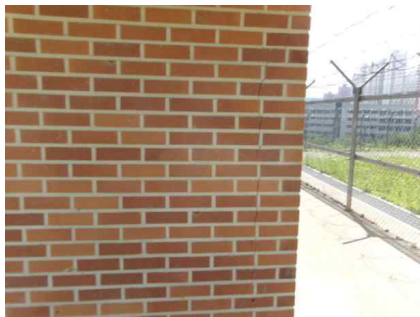
<3~4호지 검수실 외부 조적균열>
