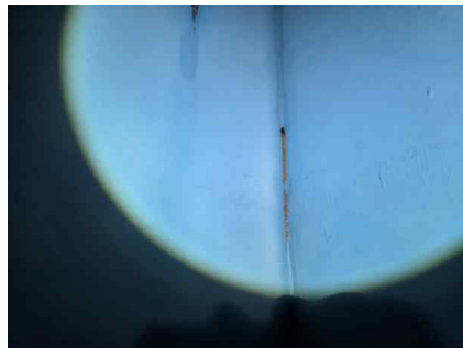
<배수지 2지 벽체 녹 발생열>
