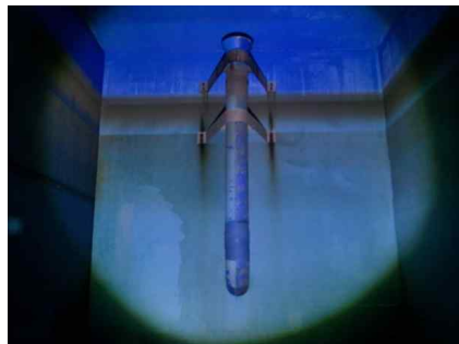
<배수지 4지 유입배관 부식>
